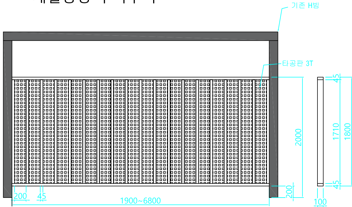
정면도 SCALE : None
