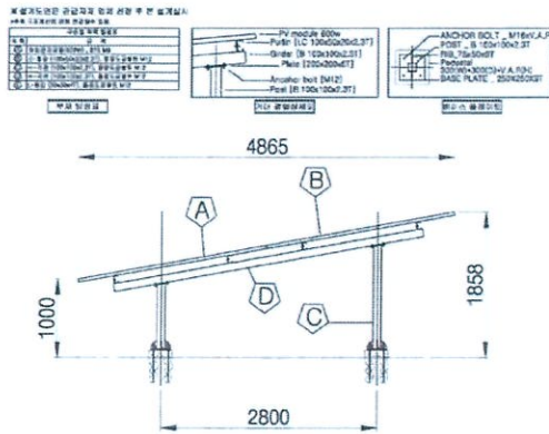
108동 정면도
