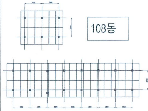
108동 배면도
